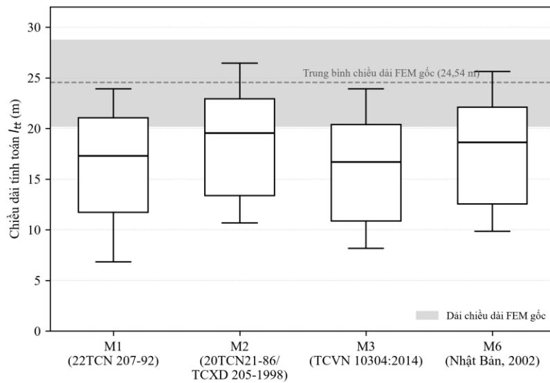
Hình 3. Phân bố chiều dài tính toán l_u của 178 cọc theo bốn phương pháp**, đối chiếu với dải chiều dài điểm ngầm giả thiết của mô hình FEM gốc.
